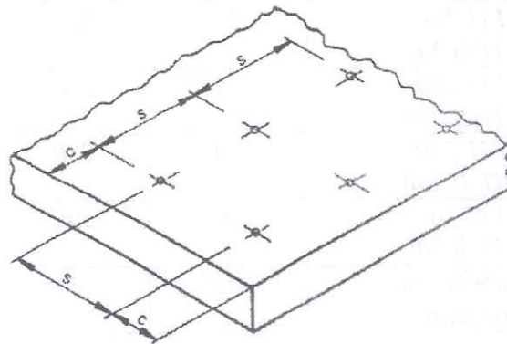
Fig. 4 Parametrii de distribuire a diblurilor pe suport s - distanta dintre axele diblurilor; c - distanta de la diblu pana la marginea suportului
